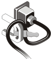
6. ábra. A tápkábel rögzítése
