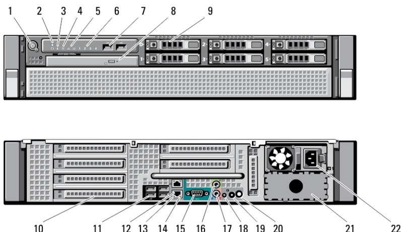
1. ábra. Elöl- és hátulnézet
